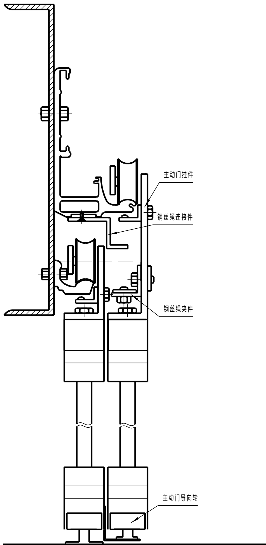
主动门挂件安装图
